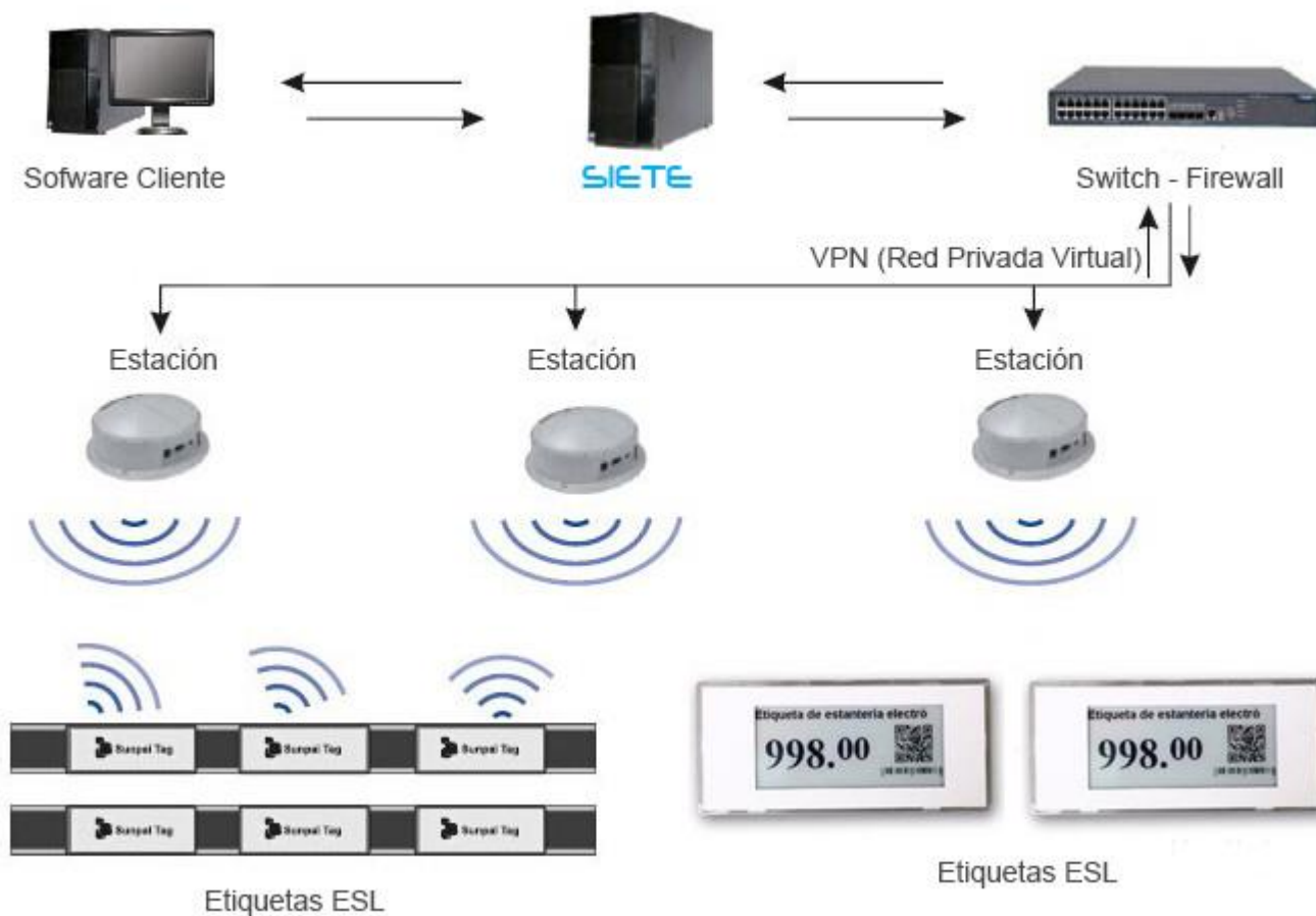
SIETE (Sistema de Etiquetado Electrónico) Diagrama Esquemático
